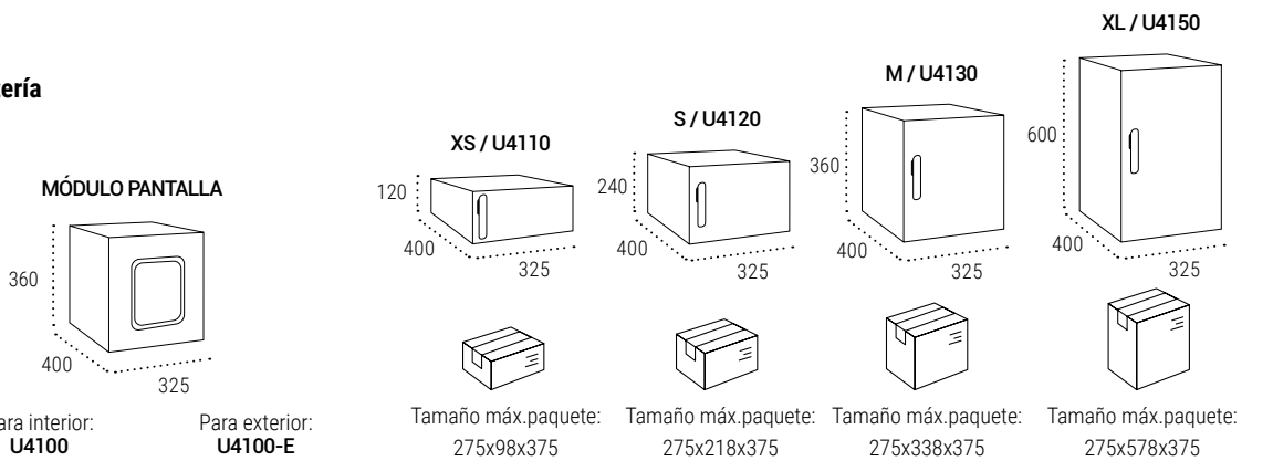
Agrupación de buzones de paquetería UNVERS DISPLAY para instalación a pared
